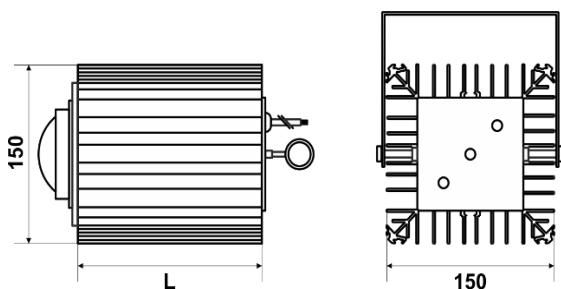
Рисунок 1. Габаритные размеры
