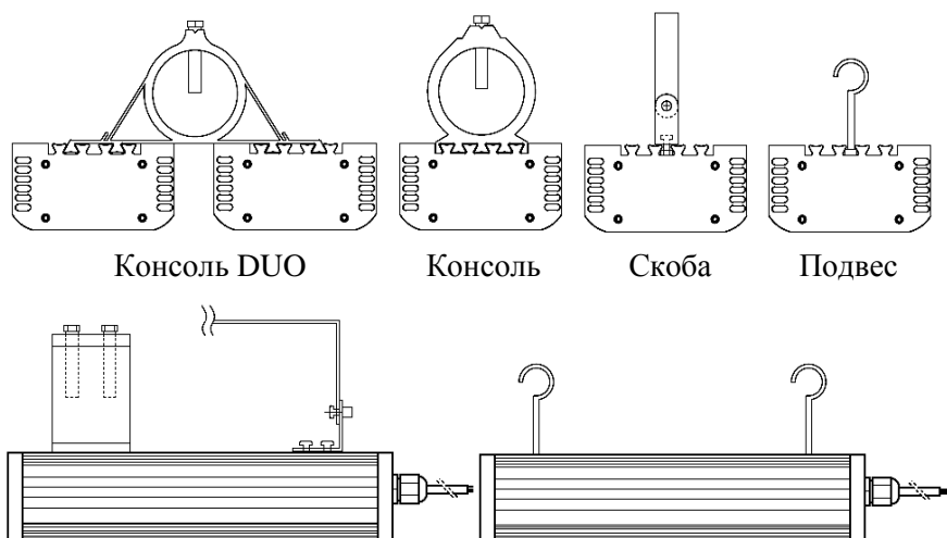
Рисунок 1. Виды креплений.
