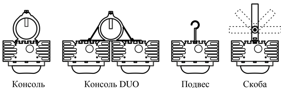
Рисунок 2. Виды креплений.
