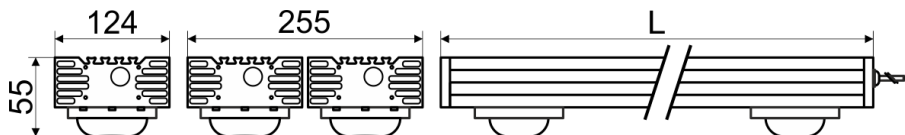
Рисунок 1. Габаритные размеры.
