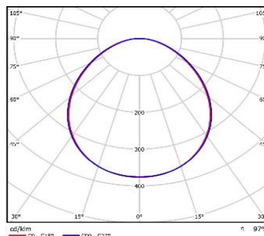
Рисунок 2. Кривая силы света
