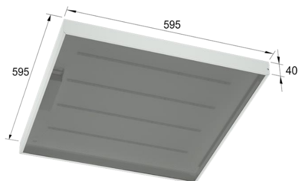
Рисунок 1. Габаритные размеры
