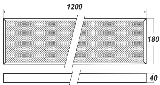
Рисунок 1. Габаритные размеры
