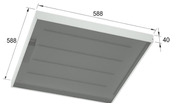
Рисунок 1. Габаритные размеры
