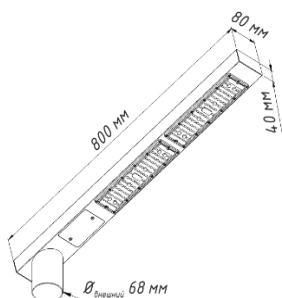
Рисунок 1. Габаритные размеры
