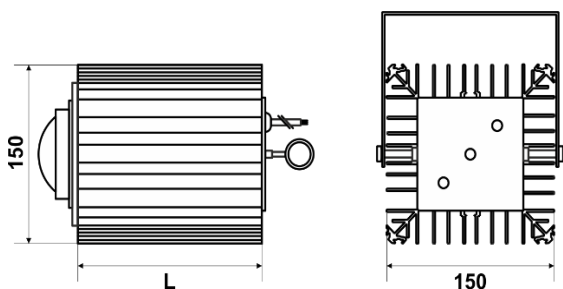
Рисунок 1. Габаритные размеры
