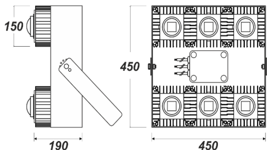
Рисунок 1. Габаритные размеры
