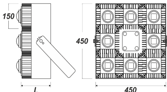
Рисунок 1. Габаритные размеры
