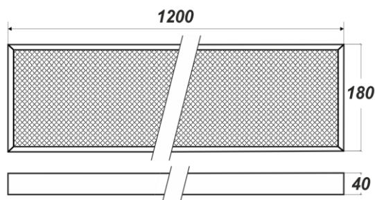
Рисунок 1. Габаритные размеры
