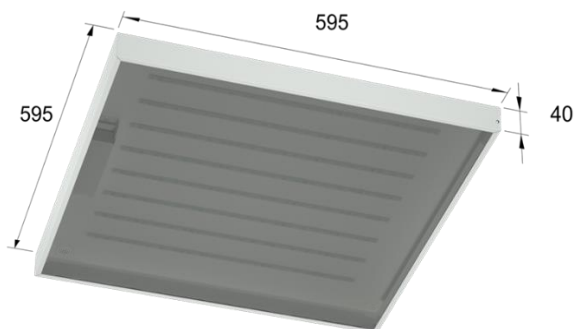
Рисунок 1. Габаритные размеры
