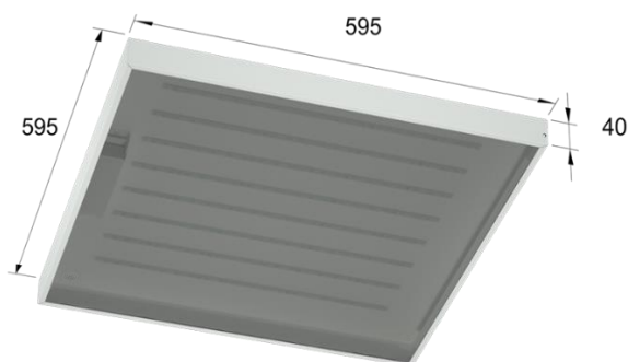
Рисунок 1. Габаритные размеры
