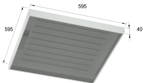
Рисунок 1. Габаритные размеры
